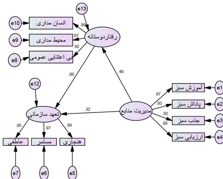
شکل ۲- مدل مفروض پژوهش (مدل میانجی) در حالت بتای استاندارد
