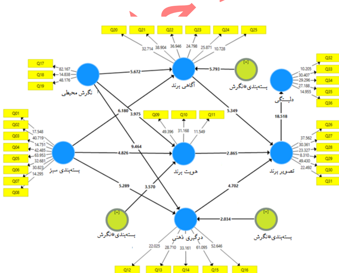
شکل ۳- مدل معادلات ساختاری در حالت آماره معناداری
